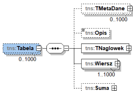
Schemat 80. Struktura elementu Tabela dla BlokDanych
