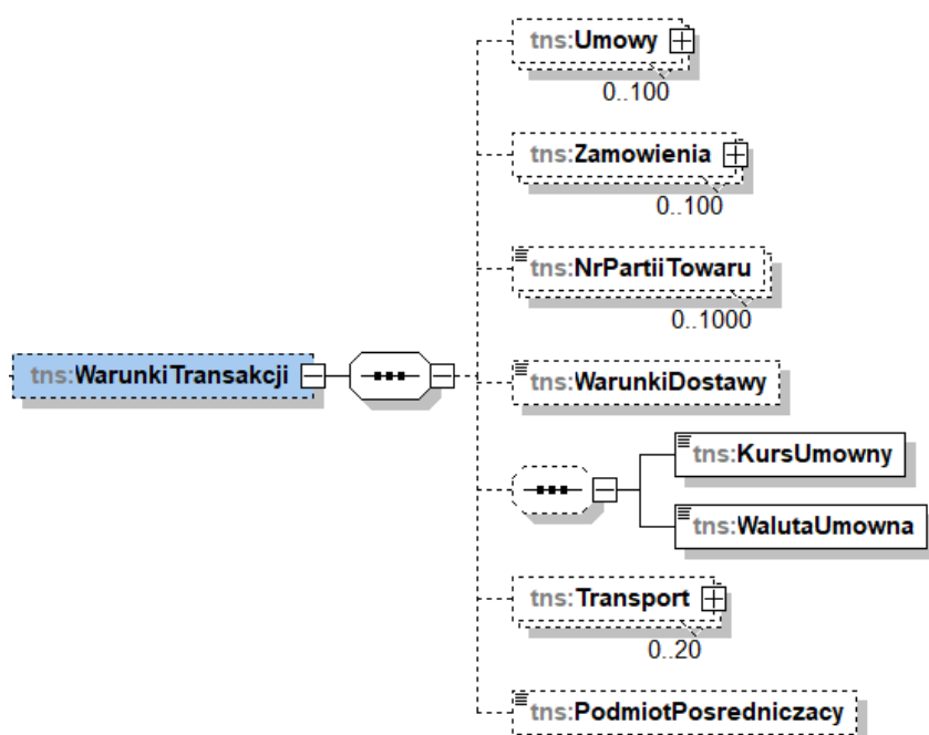
Diagram 59. Structure of the WarunkiTransakcji element for Fa
